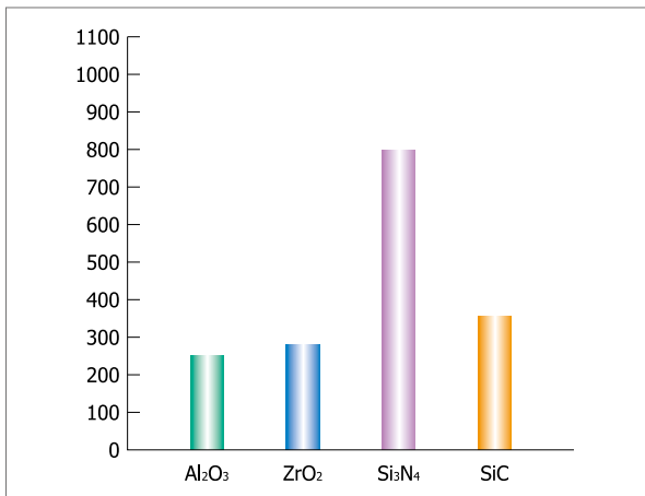
THERMAL SHOCK ( \Delta T , °C)
